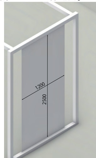
MaxSize W:1200 H:2500
